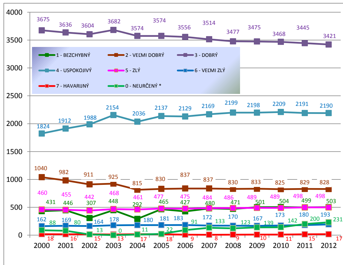
Grafické znázornenie mostných objektov z hľadiska ich stavebného stavu
