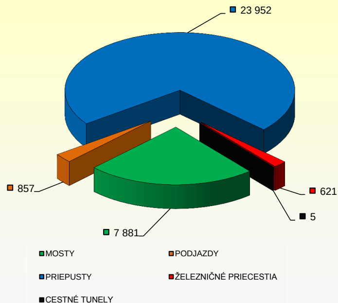
POČET CESTNÝCH OBJEKTŮV NA CESTNÝCH KOMUNIKÁCIÁCH
