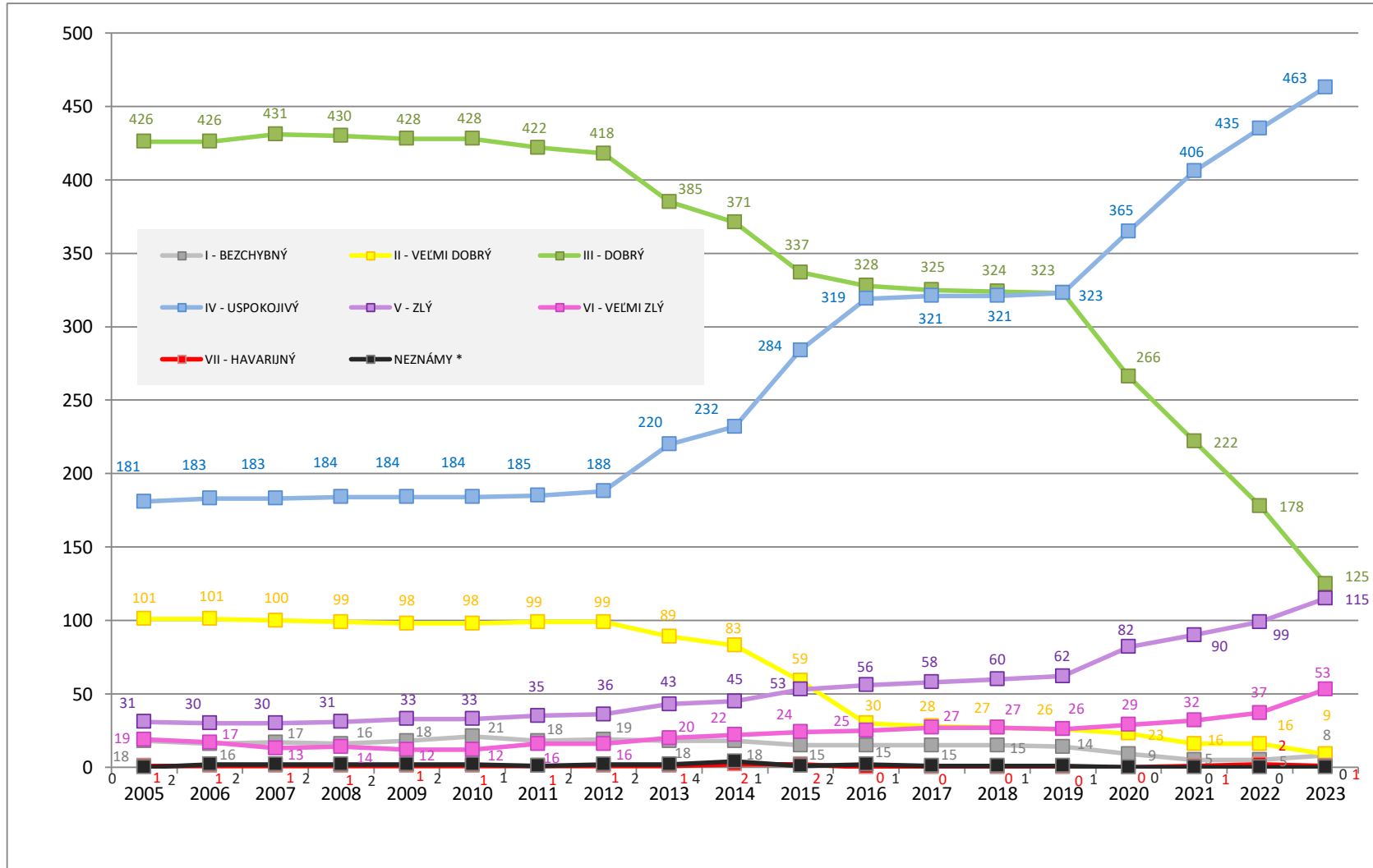
Znázornenie počtu mostov z hľadiska ich stavebno-technického stavu v správe BB SK
