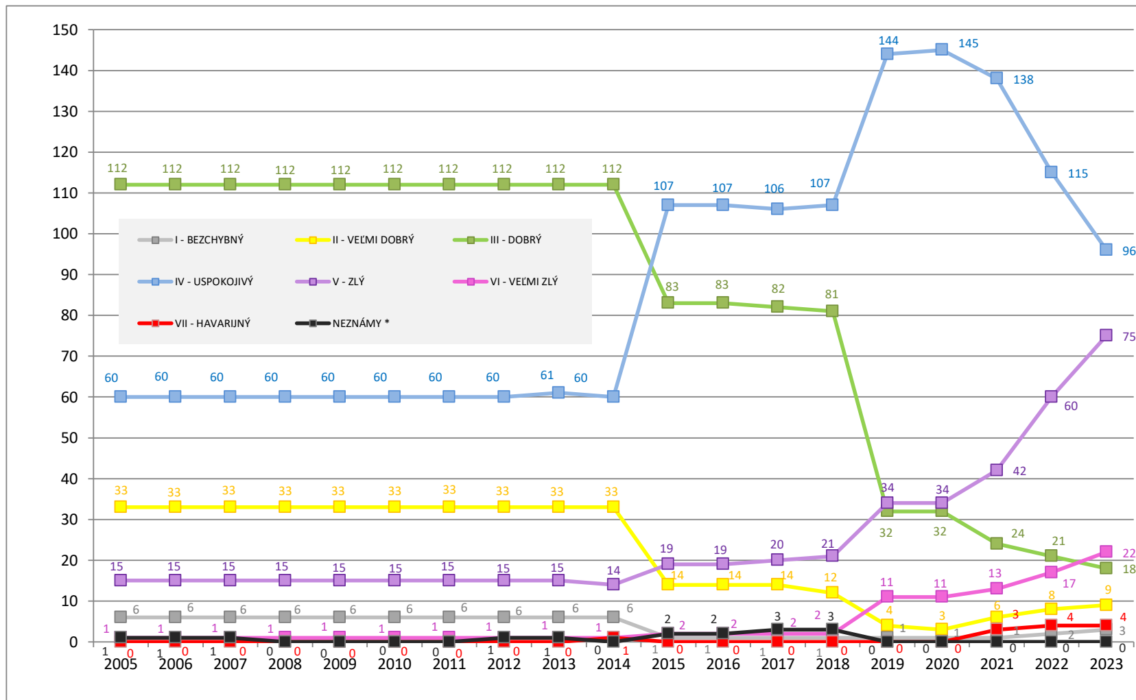
Znázornenie počtu mostov z hľadiska ich stavebno-technického stavu v správe TT SK na cestách III. triedy
